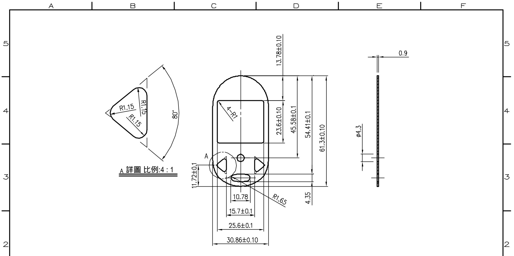
TN408LC LCD面板刀模尺寸圖
